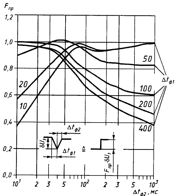
Рисунок В.2 — Коэффициент приведения F_{пр} для прямоугольных и треугольных периодических колебаний напряжения
