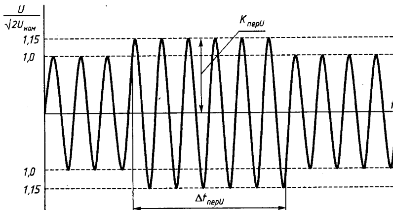
Рисунок Б.4 — Временное перенапряжение
