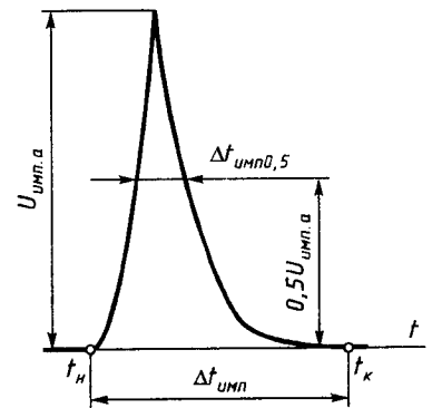
Рисунок Б.3 — Параметры импульсного напряжения
